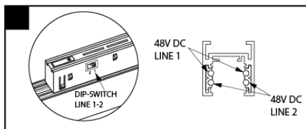
Doppia accensione – Double switch – Double interrupteur – Doppelschalter – Doble interruptor
